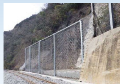
崩壊土砂防護柵 スロープガードフェンス タイプLE NETIS登録番号：HR-100008-VR
