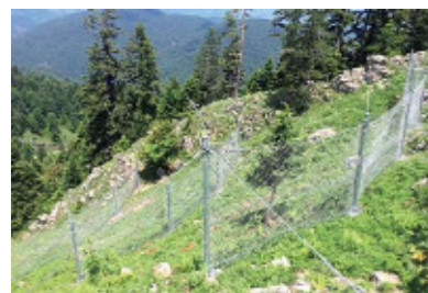
トルコで雪崩対策事業、雪崩予防柵を試験設置
